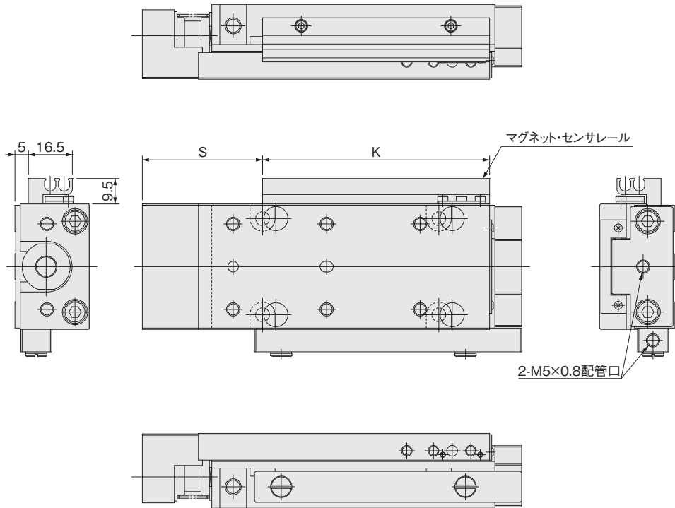
配管口方向-Rの場合
