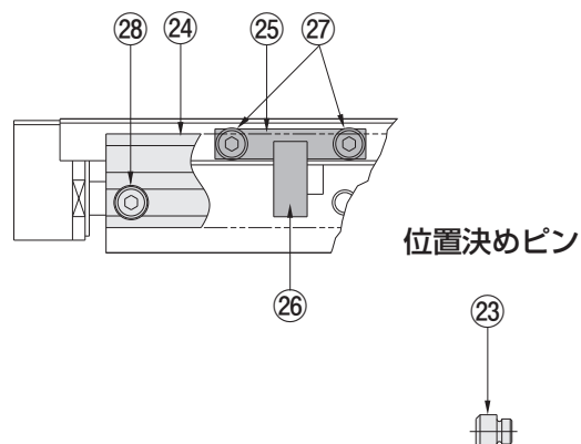
MGAPS□ (マグネット・センサレール付)
