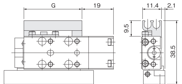
マグネット・センサーレール付の場合
