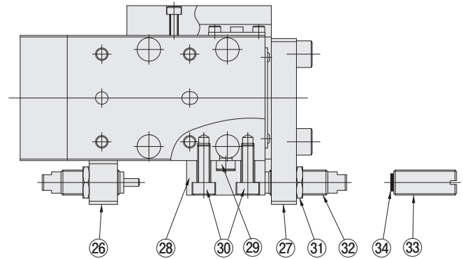
CS-MGA□10~□20 (ショックアブソーバ付)
