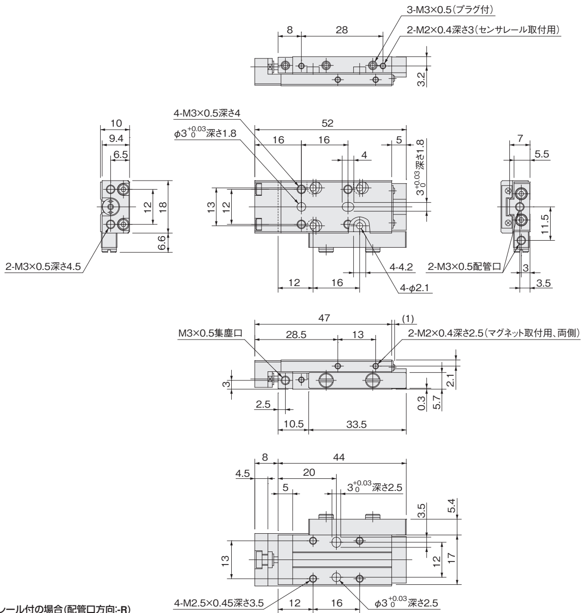
配管口方向-Rの場合
