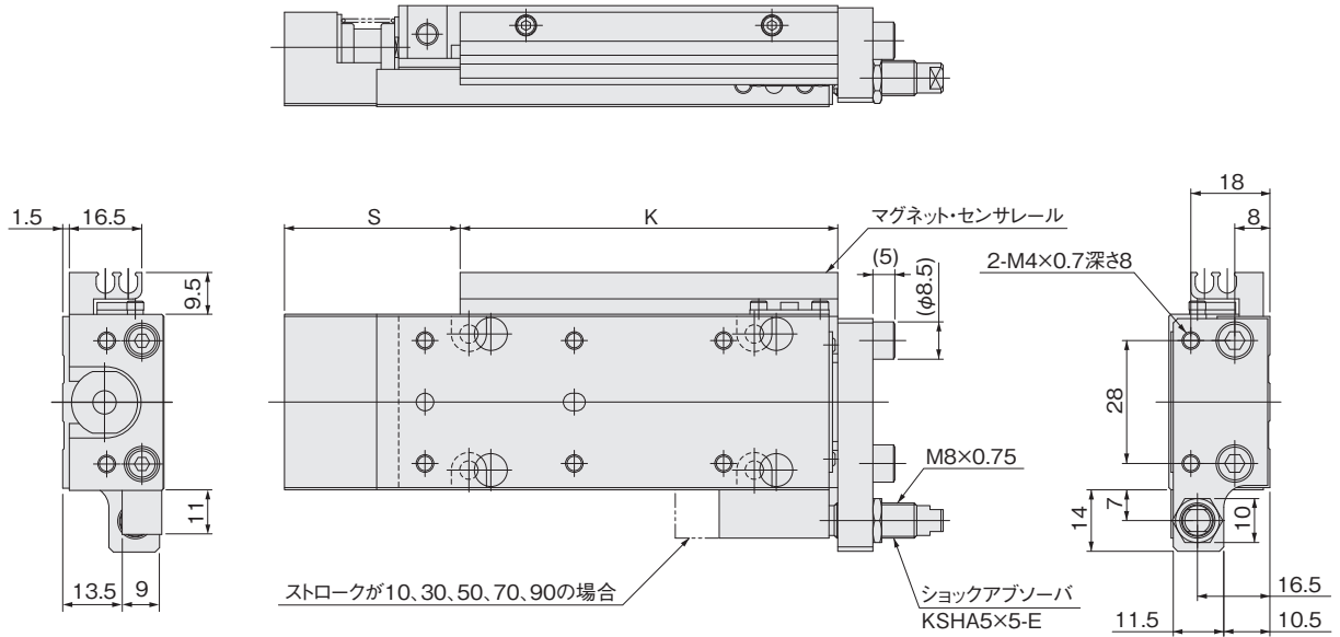
配管口方向-Rの場合
