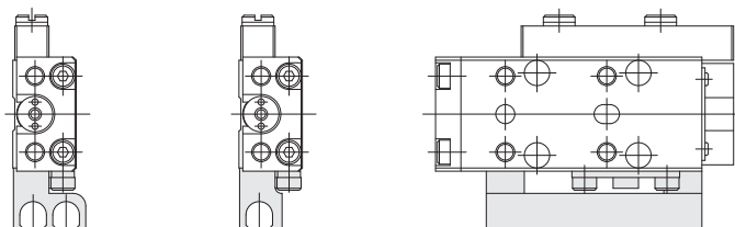
マグネット・センサレール付の場合(配管口方向:-L)
