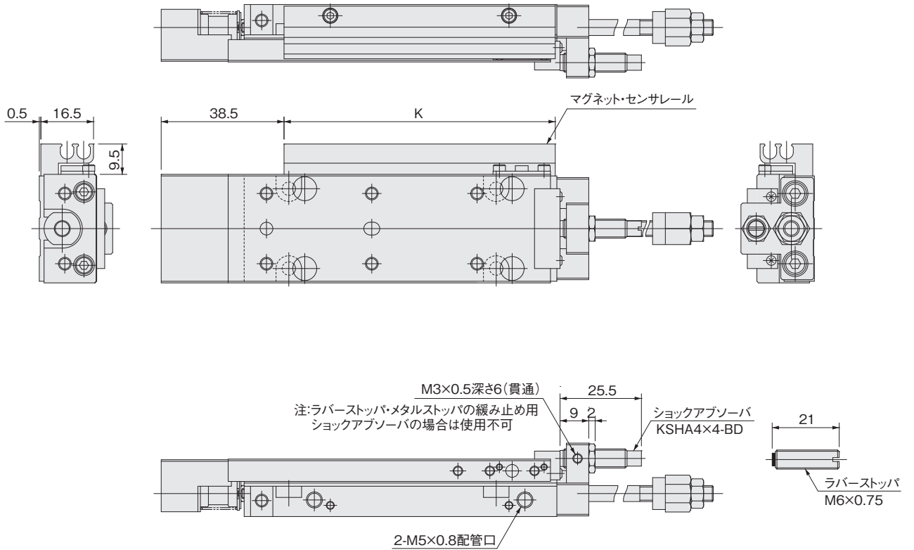
配管口方向-R,SS2の場合
