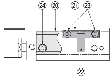
CS-MGA□10~□20 (ショックアブソーバ付)
