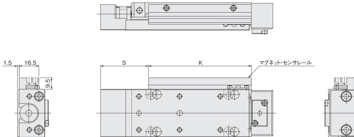
配管口方向-Rの場合
