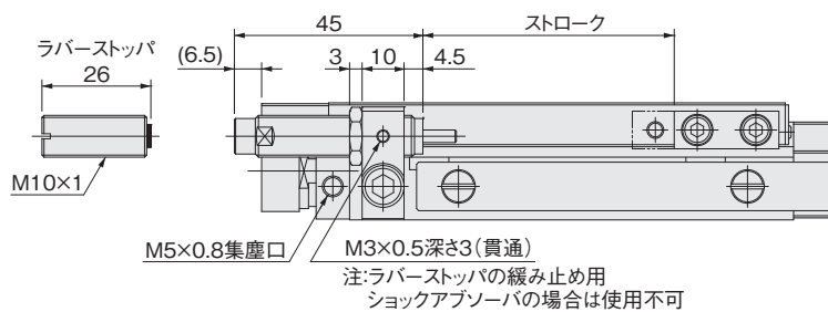
配管口方向-Lの場合 オプションなし
