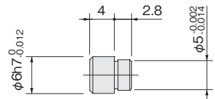
位置決めピン : -P (P-MGA3)
