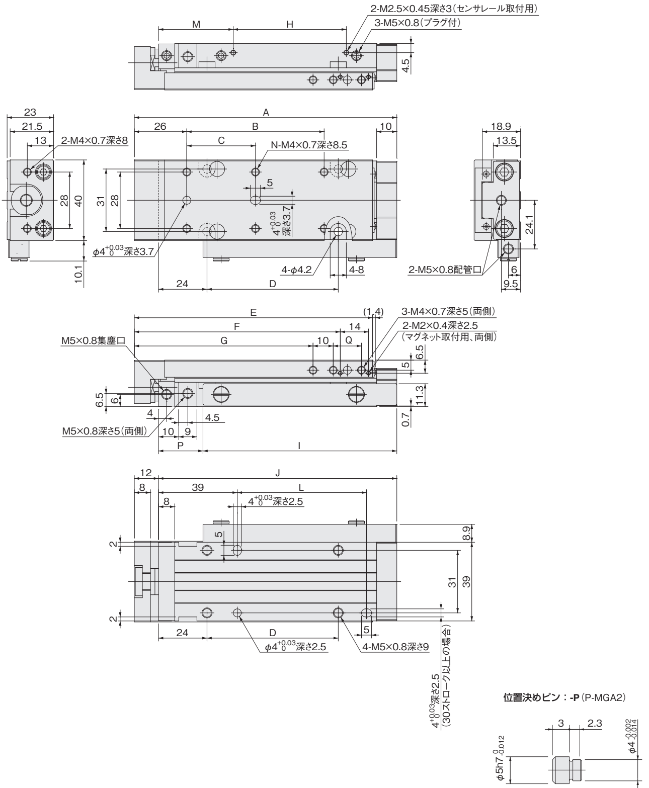
配管口方向-Rの場合
