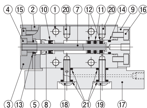
MGAL□6・8
