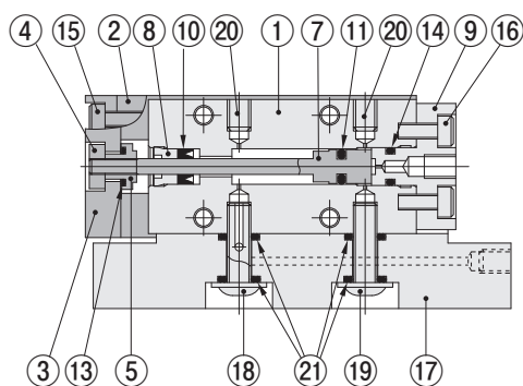
MGAL□10
