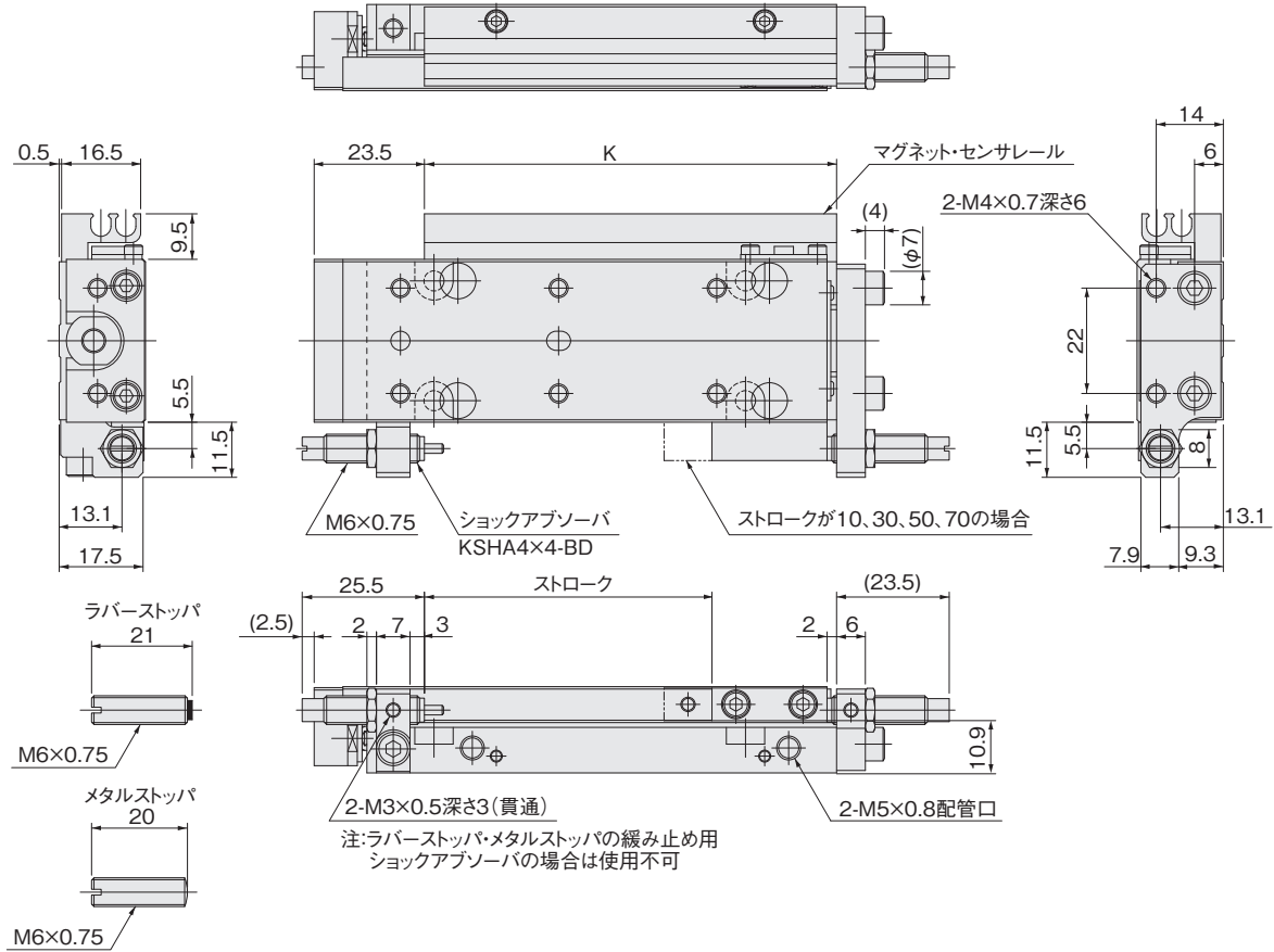
配管口方向-Lの場合
