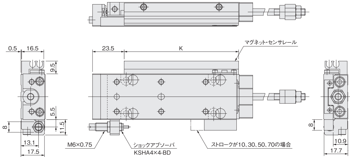
配管口方向-Rの場合
