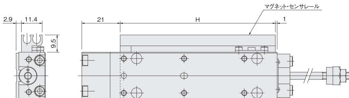
配管方向-Rの場合
