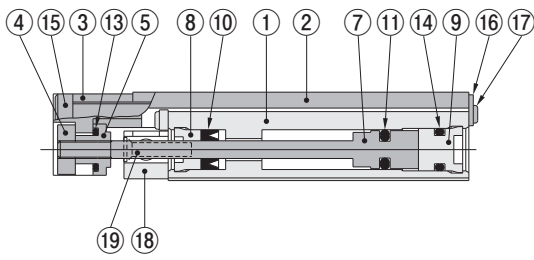
CS-MGA□10~□20
