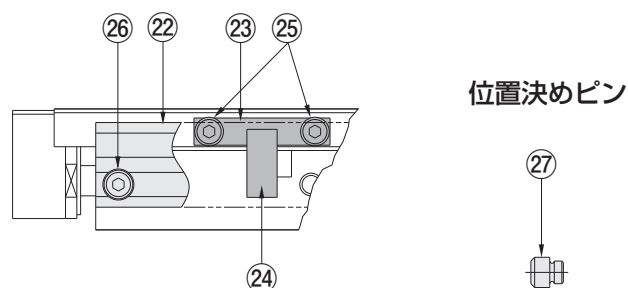
MGALS□ (マグネット・センサレール付)
