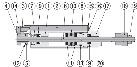
MGAP□6・8・10
