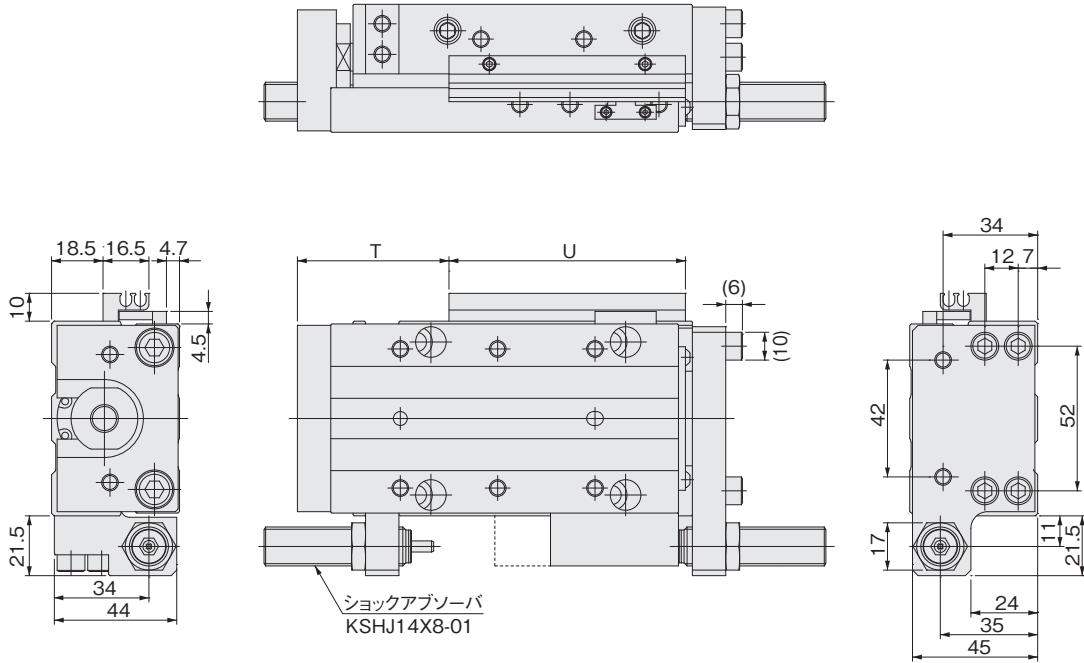
配管口方向-Rの場合
