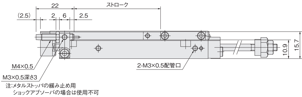
配管方向:-Lの場合
