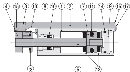
MGA□25~□32
