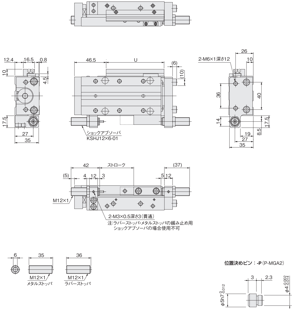
配管口方向-Rの場合
