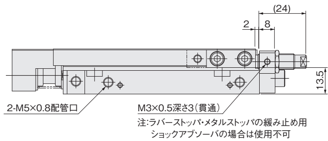
配管口方向-Lの場合
