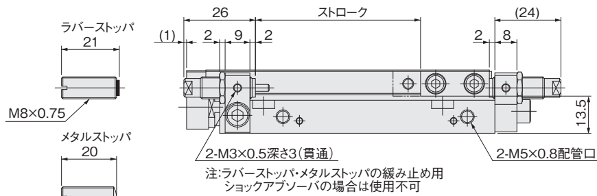
配管口方向-Lの場合
