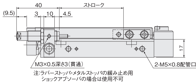
配管口方向-Lの場合
