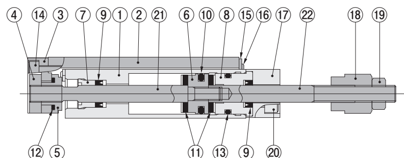
MGAP□12・16・20
