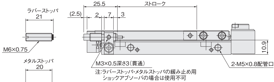
配管口方向-Lの場合
