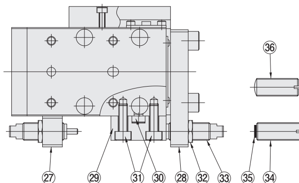
MGA□10~□32 (ショックアブソーバ付)
