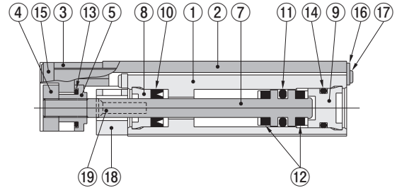
CS-MGAS□ (マグネット・センサレール付)
