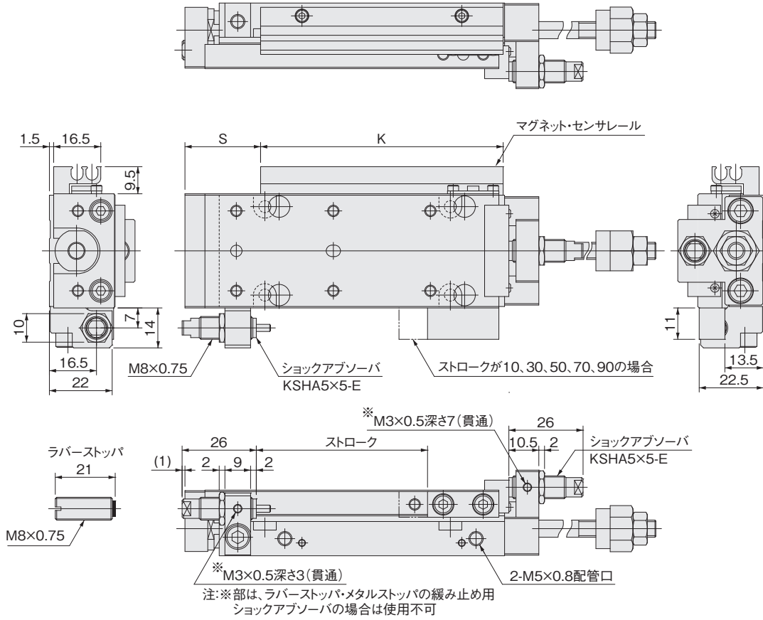
配管口方向-Rの場合
