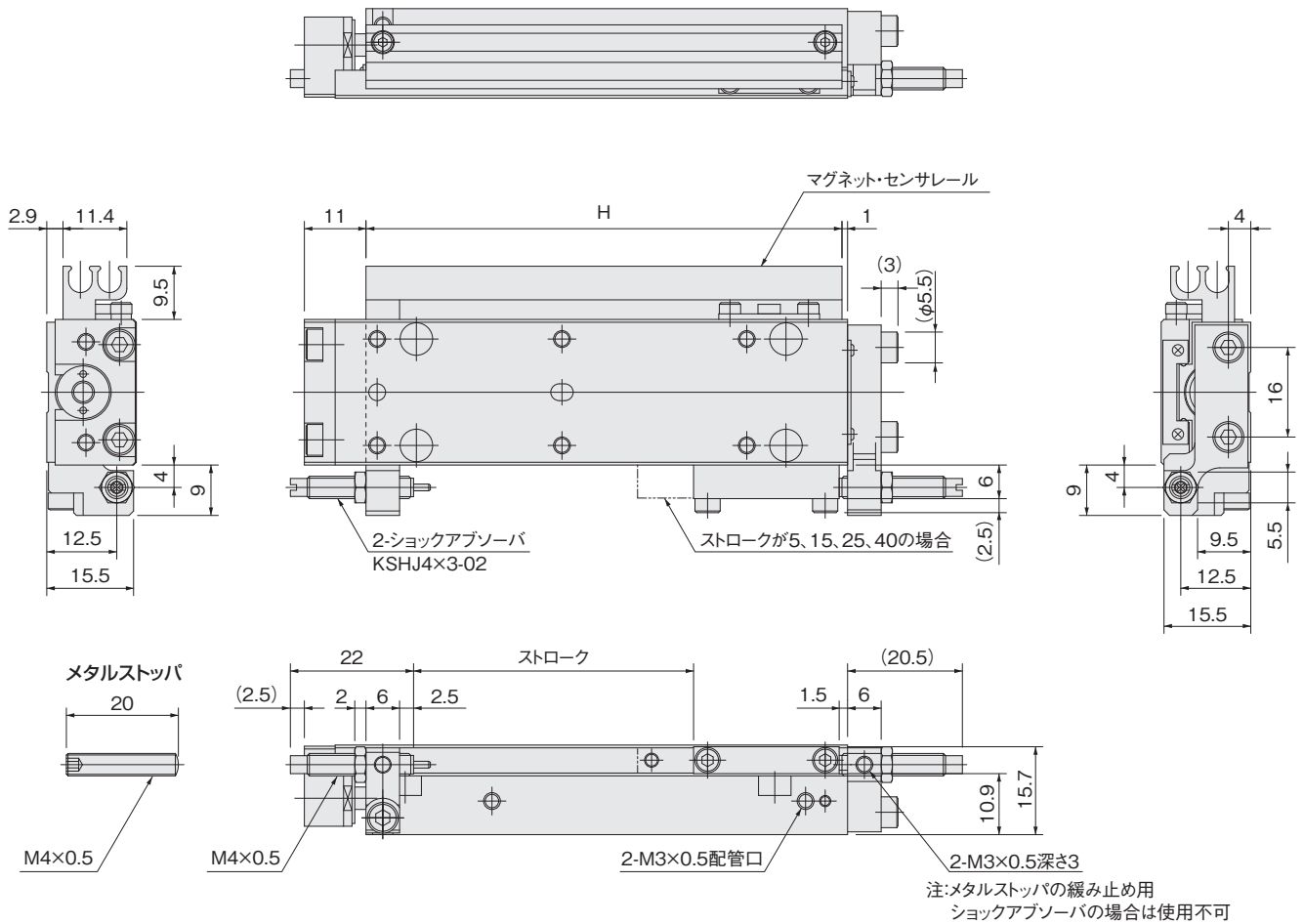
配管方向-Rの場合
