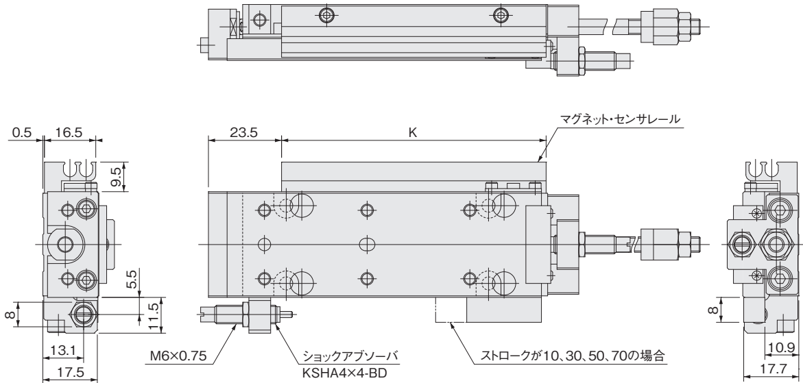
配管口方向-R,-SS2の場合
