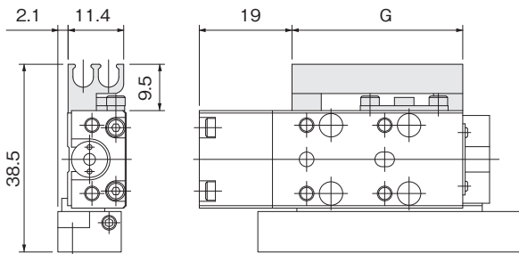
マグネット・センサレール付の場合
