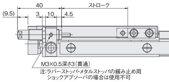
配管口方向-Lの場合
