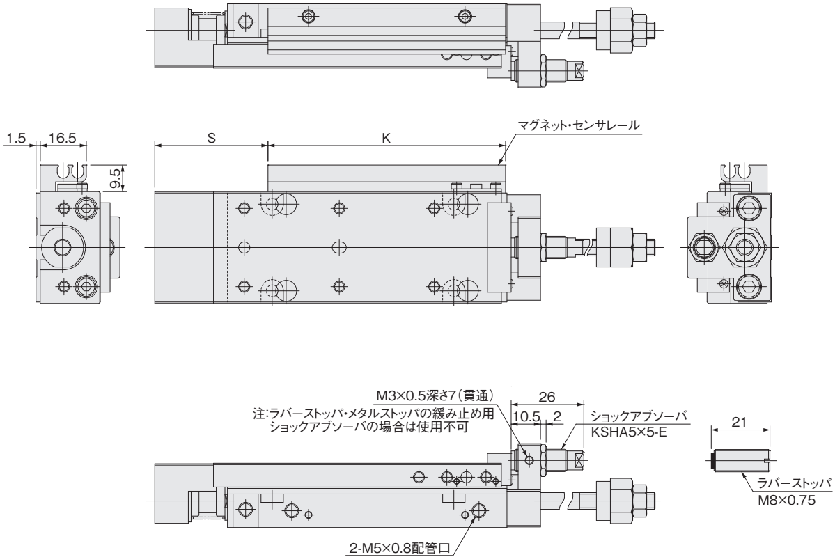
配管口方向-Rの場合
