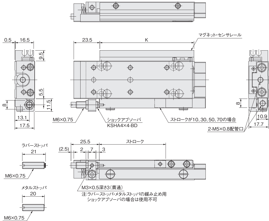
配管口方向-Lの場合
