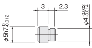
位置決めピン: -P (P-MGA2)
