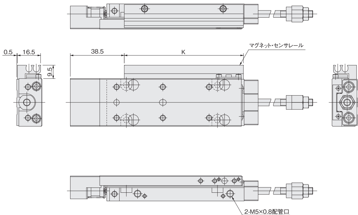
配管口方向-Rの場合
