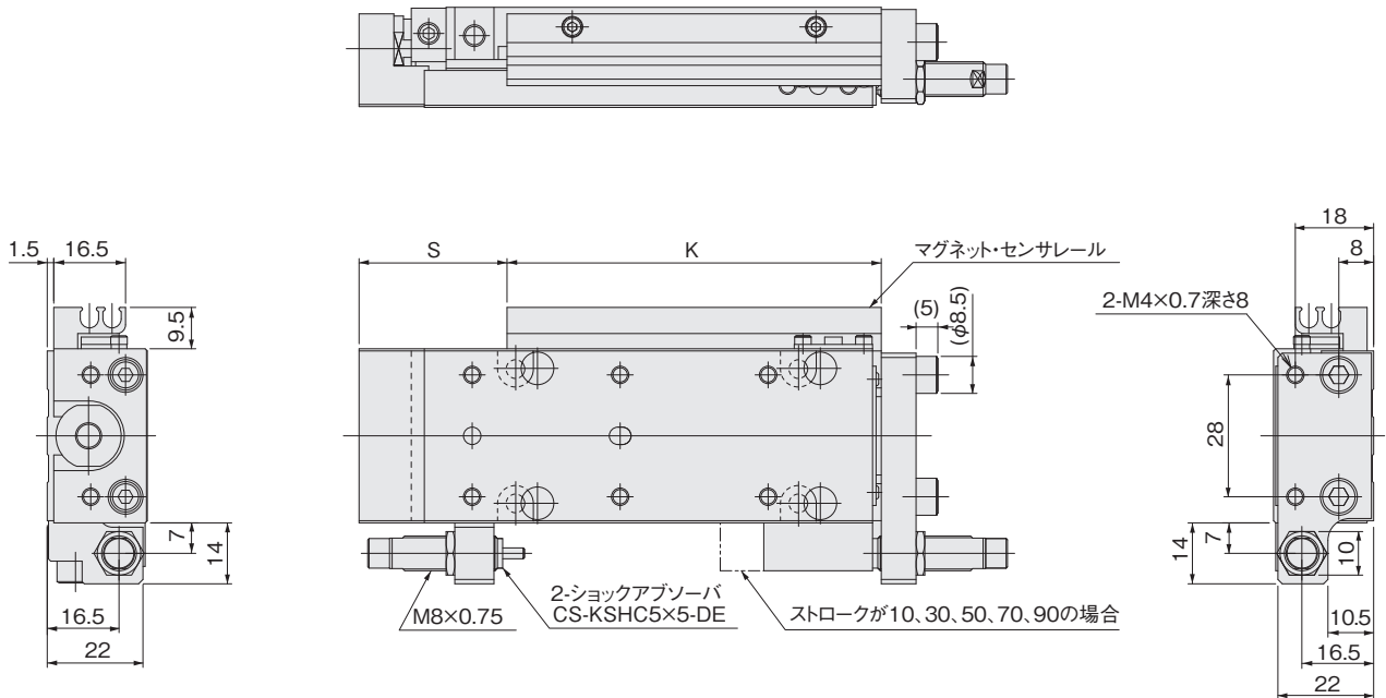
配管口方向-Rの場合
