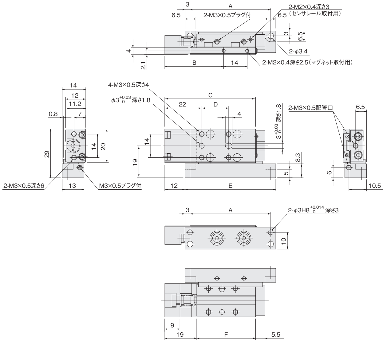
マグネット・センサレール付の場合
